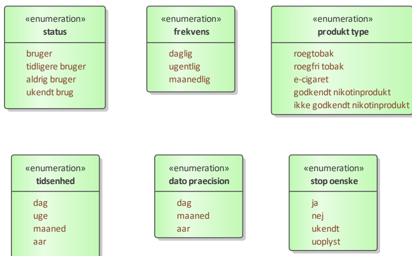
Figur 3 Informationsmodellens enumerationer
